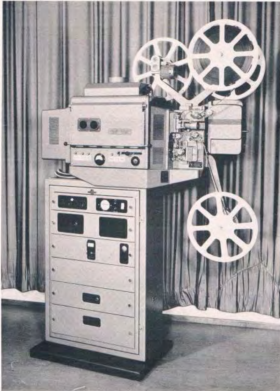
Zweibandprojektor 16/16 für 16-mm-Schmalfilm Typ BAUER-SELECTON-II-0, auf Siemens-Verstärkergestell Bauart Fernsehen
