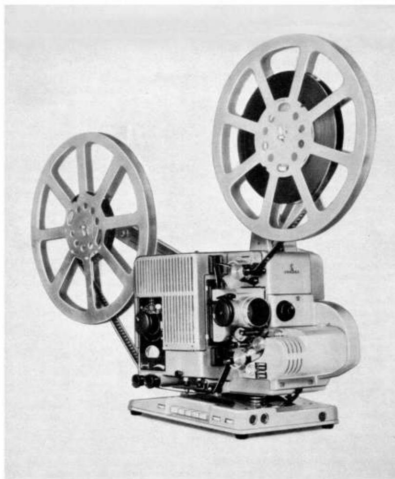
Siemens-Tonfilm-Projektor „2000“ für Lichtton-Wiedergabe, Sockelverstärker, Ausführung SL.
