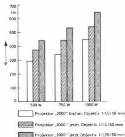
Bild 6. Nutzlichtstrom beim Projektor „2000“, gemessen mit Zweiflügelblende; Mittelwert aus 9 Meßpunkten des ausgeleuchteten Bildfensters
