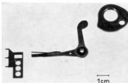
Bild 4. Dreizahngreifer, Greiferschalthebel und Schaltkurve aus dem Siemens-Projektor „2000“
