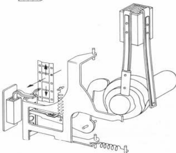
Bild 3. Schmierstoffversorgung des Filmschaltwerks
