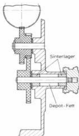
Bild 2. Nachwickelwelle mit selbstschmierenden Sinterlagern
