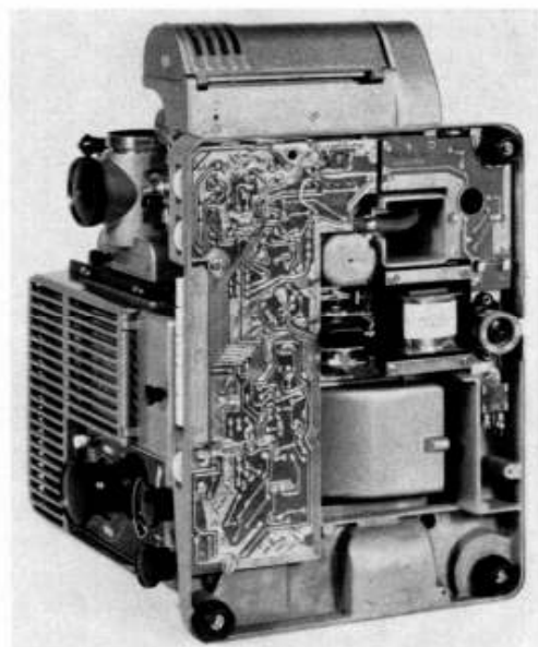
Bild 7. Transistor-Sockelverstärker; Ansicht von unten (ohne Bodenblech)
